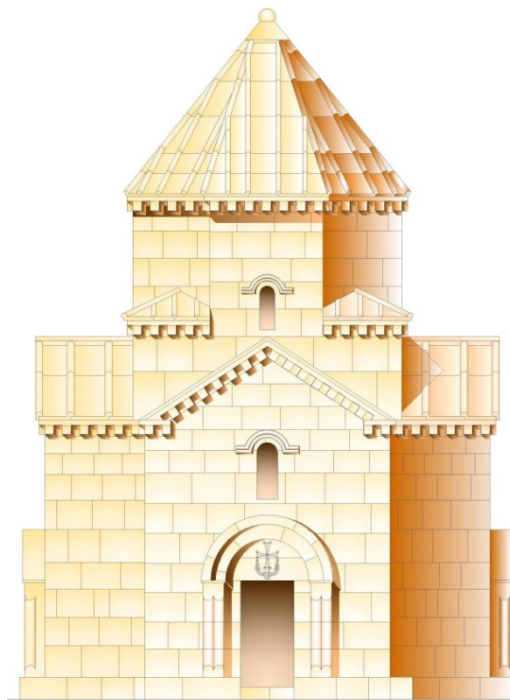
ԱՐԵՎԱՏՅԱՆ ՃԱԿԱՏ Մ 1:50
